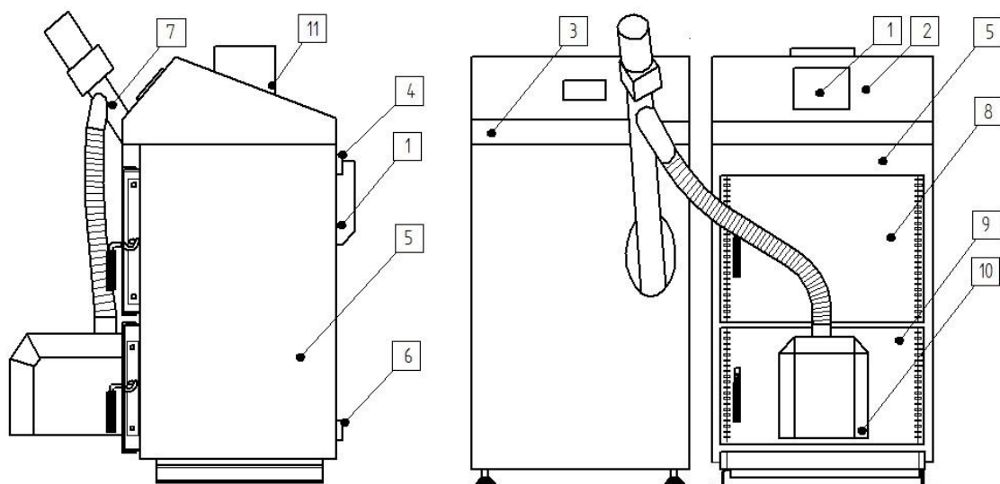
rys.1 Schemat budowy kotłów PERIKS OPTIMA BIO
