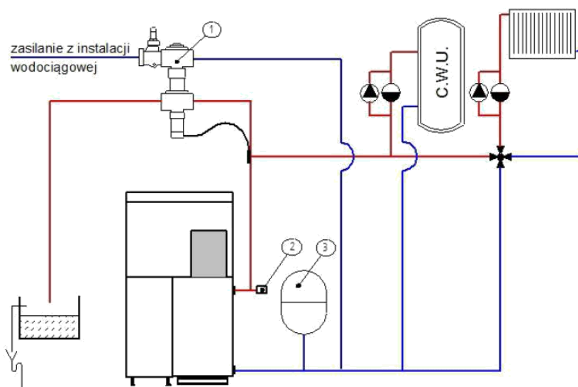
1- zabezpieczenie termiczne 5067 2 - zawór bezpieczeństwa 3 - przeponowe naczynie wzbiornicze
