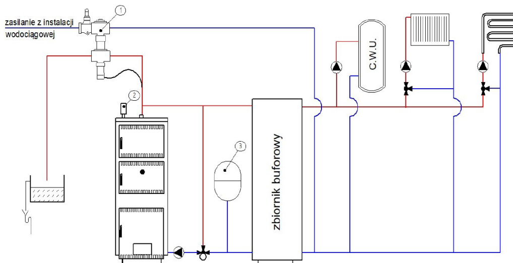
1- zabezpieczenie termiczne 5067 2 - zawór bezpieczeństwa 3 - przeponowe naczynie wzbiornicze
