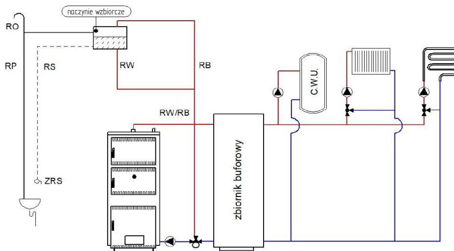
RO-rura odpowietrzająca RB-rura bezpieczeństwa RW-rura wzbiornicza RP-rura przelewowa RS-rura sygnalizacyjna ZRS-zawór rury sygnalizacyjnej
